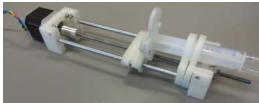
Figura N.º 8. Bomba para jeringa.
