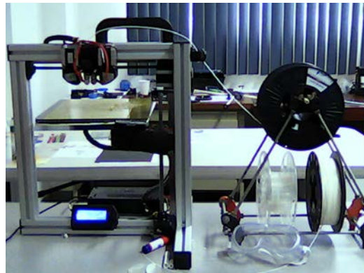
Figura N.º 2. Equipo de impresión 3D utilizado para el presente estudio. El modelo Félix Printers 3.1 trabaja con el método por extrusión fundida y es de arquitectura abierta. Especificaciones en FélixPrinters, s.f.
