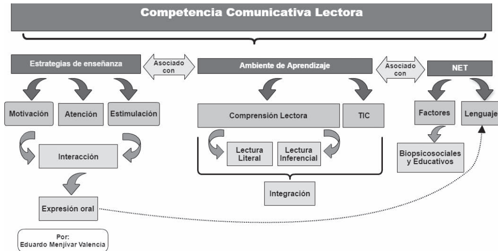
Figura 1. Red semántica
